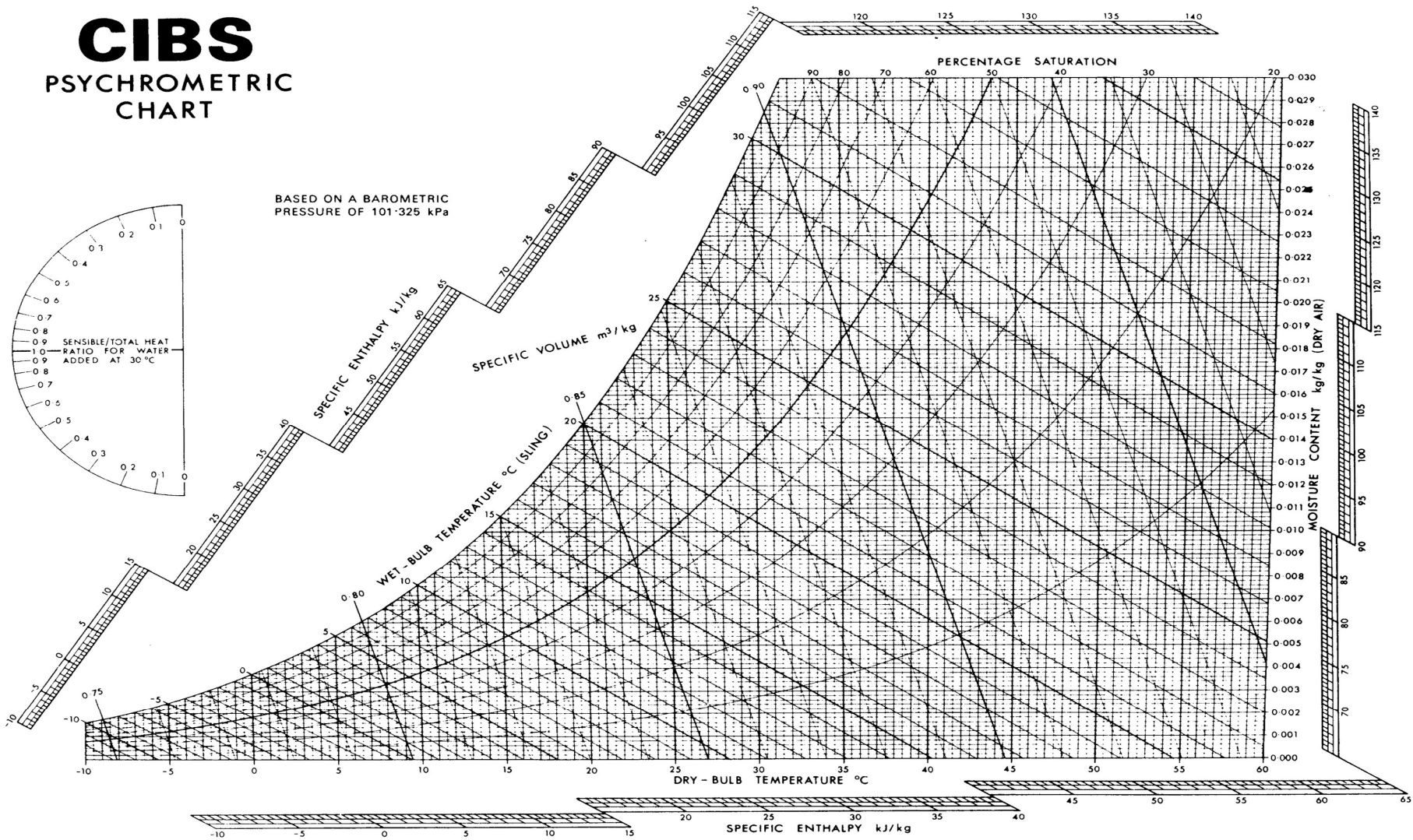
Σχήμα ΨΥ-3. Ψυχομετρικός χάρτης
